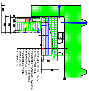
SCHNITT C-C' - UMFANGSWANDAUFBAU M=1:10
